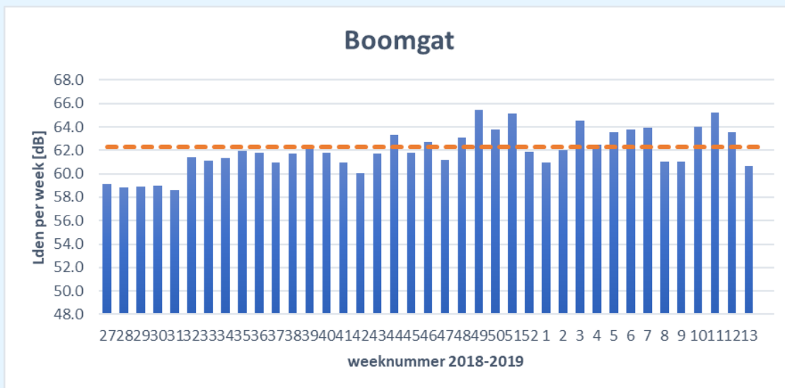
figuur 18: verloop L den wegverkeer per week voor locatie Boomgat
