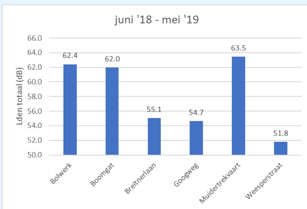
figuur 16: gemiddelde geluidsniveaus wegverkeer over de totale meetperiode
