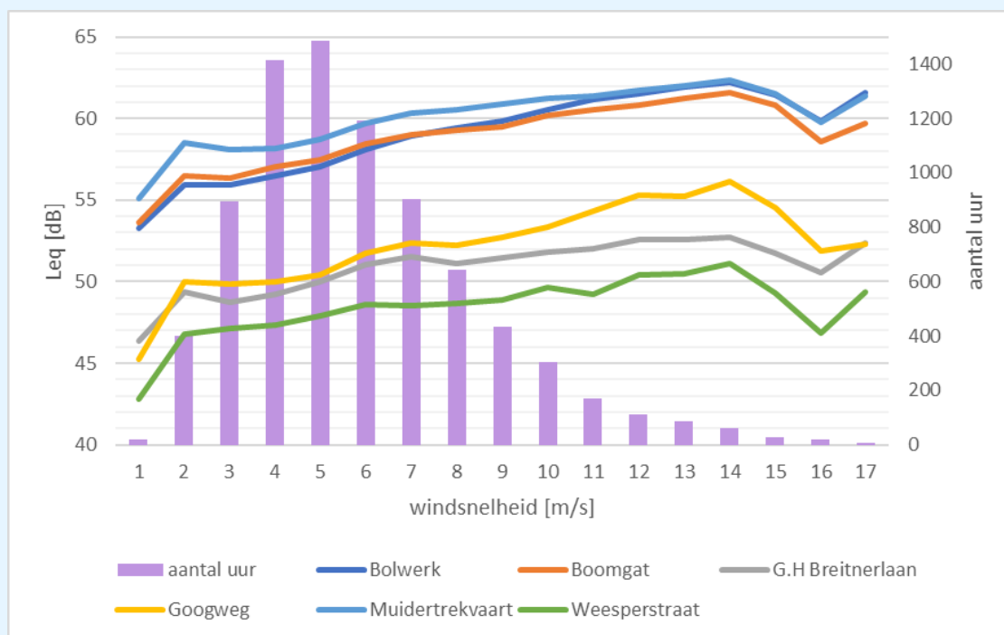
figuur 9: Gemiddelde gemeten geluidsniveau ( L_{eq} ) en aantal uur per windsnelheid over de totale meetperiode
