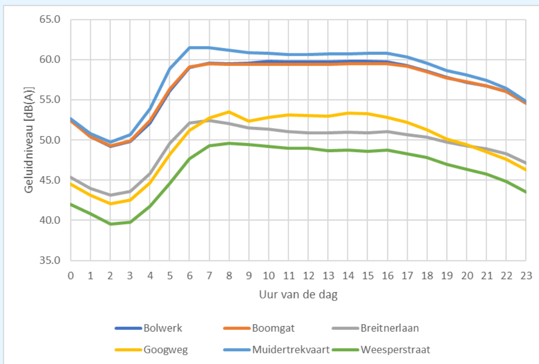
figuur 14: verloop van geluidsniveau vanwege wegverkeer over een dag
