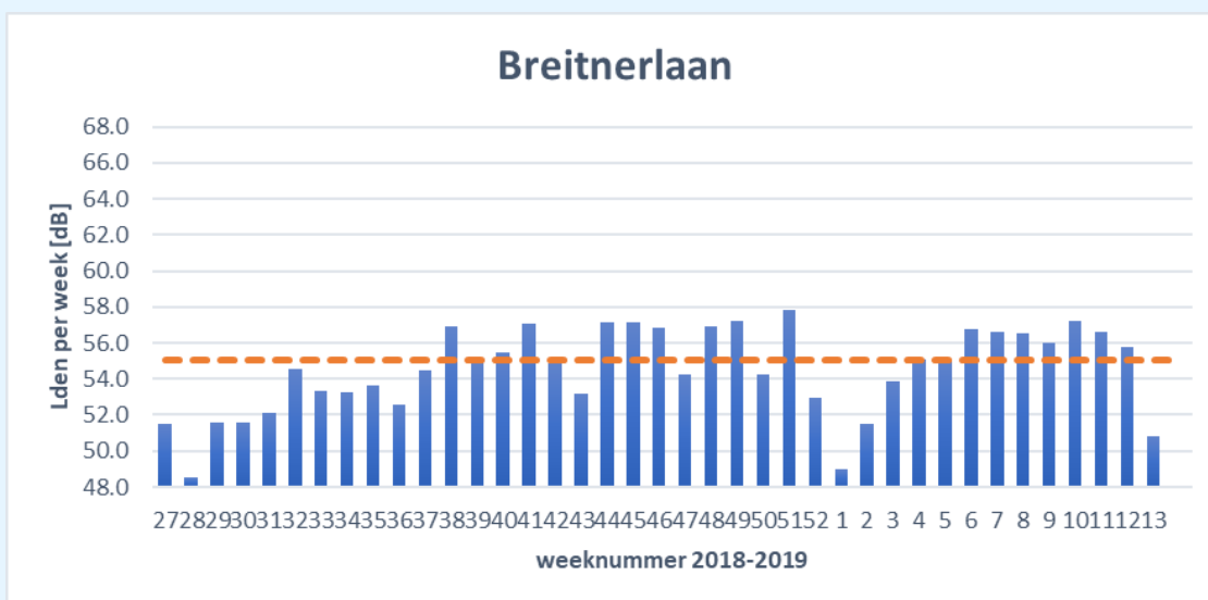
figuur 19: verloop L den wegverkeer per week voor locatie G.H. Breitnerlaan
