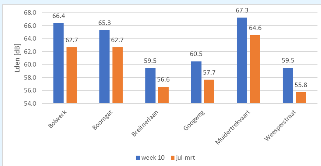
figuur 24: Gemeten L_{den} over de meetperiode juli-maart en het gemeten L_{den} van week 10
