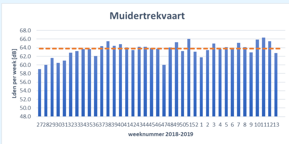
figuur 21: verloop L den wegverkeer per week voor locatie Muidertrekvaart
