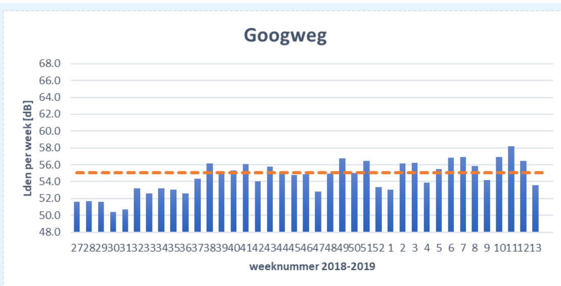
figuur 20: verloop L den wegverkeer per week voor locatie Googweg
