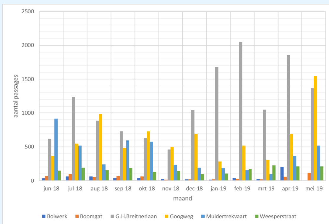
figuur 10: getelde vliegtuigpassages per maand voor alle meetlocaties
