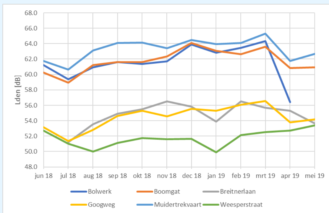
figuur 13: verloop van L_{den} voor wegverkeer over de gehele meetperiode
