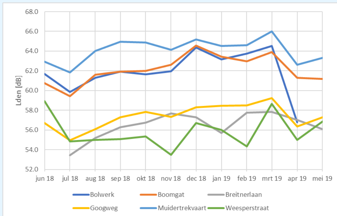
figuur 4: verloop van de gemeten totaalniveaus in Lden
