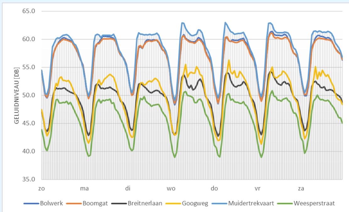
figuur 15: verloop van geluidsniveau van wegverkeer over de dagen van de week
