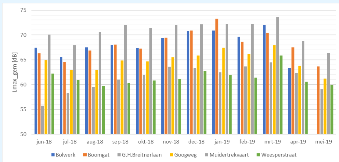
figuur 12: gemeten maximale geluidniveaus per maand vanwege het vliegverkeer
